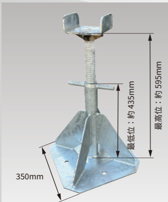
ガルバニズドリットジャッキ 品番：SPO-YBT-RACK 税込：22,000円 (税別：20,000円)
