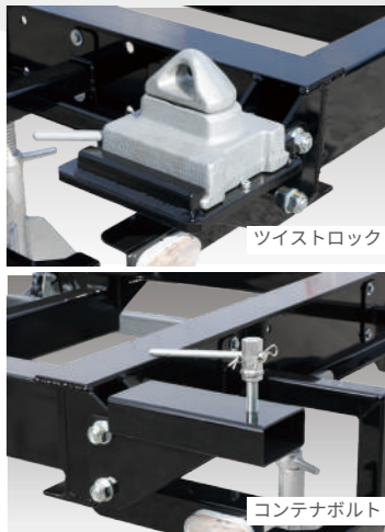
※リジットジャッキ設置例
