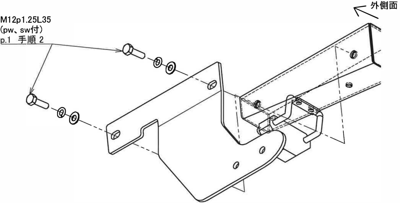
ステー取付図 ※左側を示す
